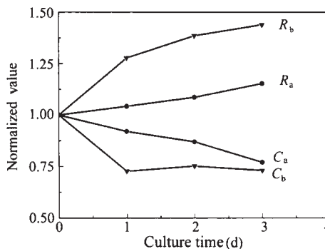
图 5 f=3981\text{ Hz} 时钛电极表面阻抗标准化元件值随培养时间的变化
