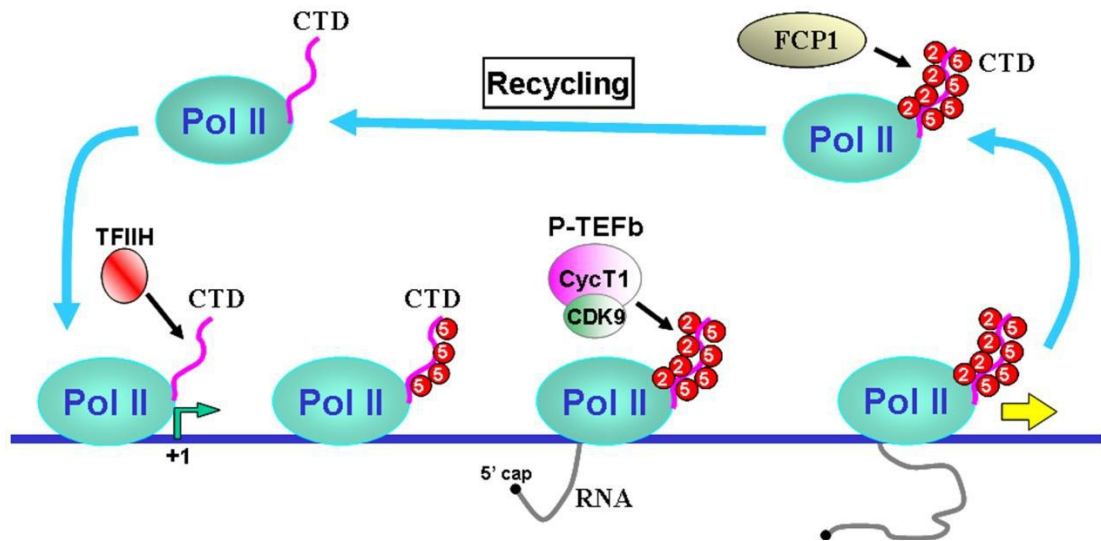
图 1.2 RNA Pol II CTD 磷酸化循环 [33]
