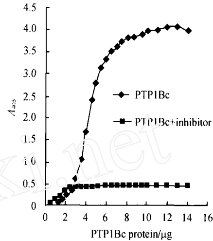
图 5 PTP1Bc 酶活分析
