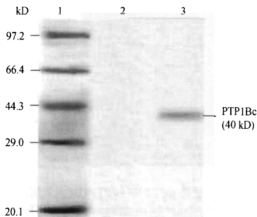
图 4 重组蛋白的 Western blotting 分析
