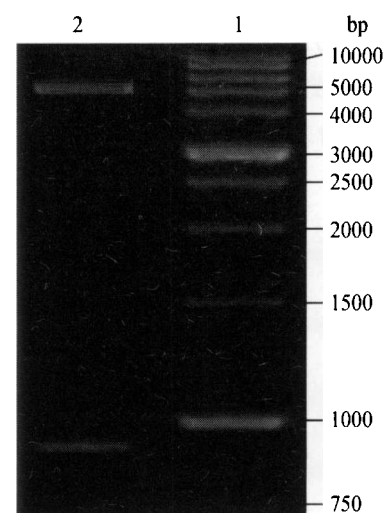
图 2 重组质粒 pET-22b(+)/PTP1Bc 的酶切鉴定
