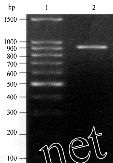
图 1 PCR 产物电泳图(1.7%琼脂糖)
