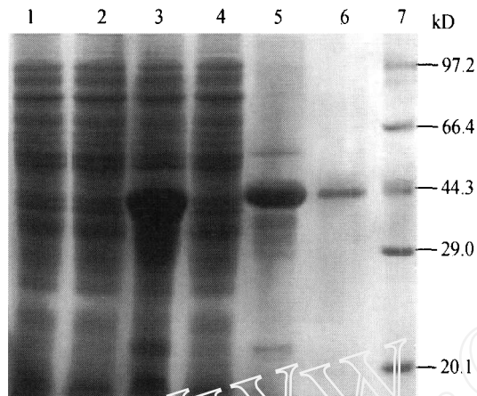
图 3 表达蛋白的 SDS-PAGE 分析
