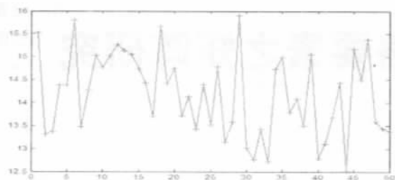
图4 t-APARCH(1,1)模型的 Hong & Li 统计量 \hat{Q}(j) 直观图 (横轴表示滞后阶数,纵轴表示统计量的值)
