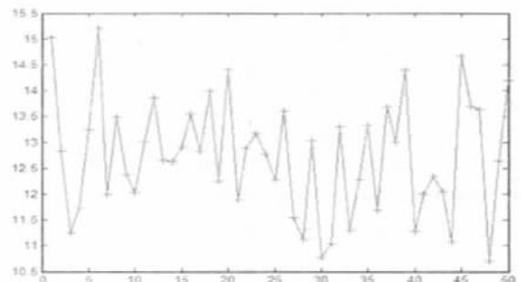
图3 GARCH(1,1)模型的 Hong & Li 统计量 \hat{Q}(j) 直观图 (横轴表示滞后阶数,纵轴表示统计量的值)
