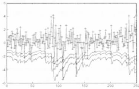
图1 GARCH(1,1)模型在 VaR 水平分别为1%、5%与 10%时的 回顾测试结果。VaR 例外数 N=3、9、17。
