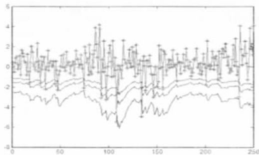
图2 t-APARCH(1,1)模型在 VaR 水平分别为 1%、5%与10%时的 回顾测试结果。VaR 例外数 N=2、10、19。
