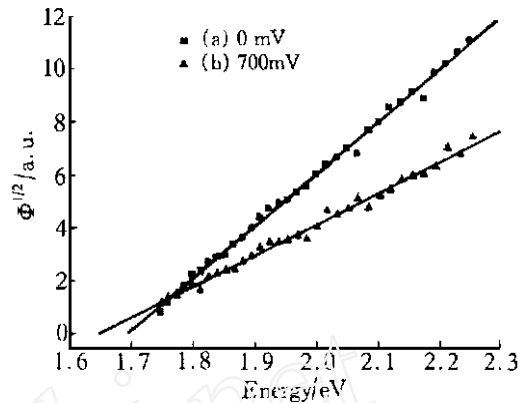
图 4 部分氧化态 PANI 的 \phi^2 和 h 的关系图
