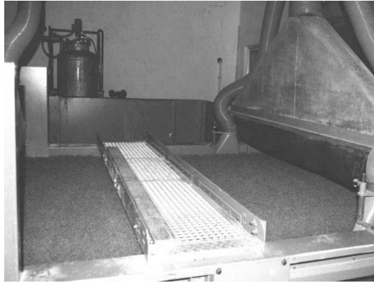
图四 铺片
