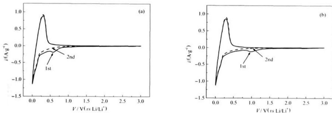
图3 MCMB电极在不同电解液中的循环伏安图
