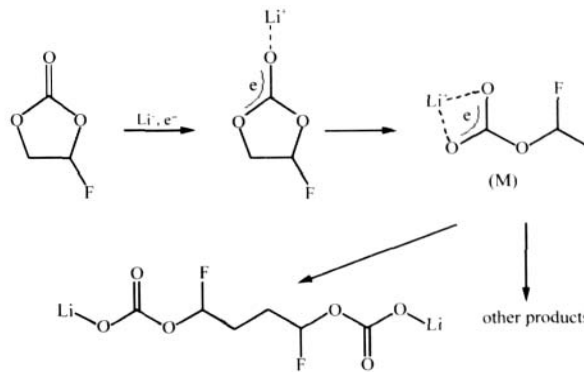
图9 FEC 的反应机理 Fig.9 The reaction mechanism of FEC
