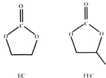
图8 EC 和 FEC 的化学结构式 Fig.8 Chemical structures of EC and FEC
