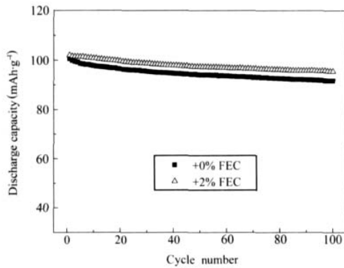
图2 室温下以0.5C倍率充放电的 \text{LiMn}_2\text{O}_4/\text{Li} 电池的循环性能曲线
