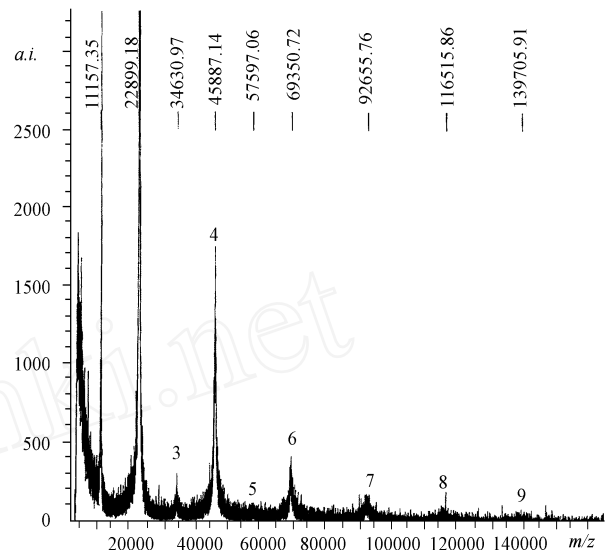
图4 NE2 蛋白的 MALDI-TOF-MS 图
