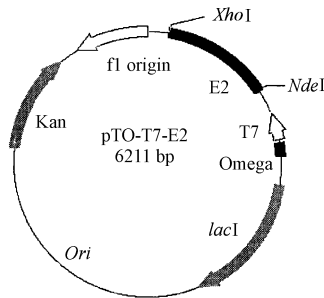
图 1 pTO-T7-E2 质粒图
