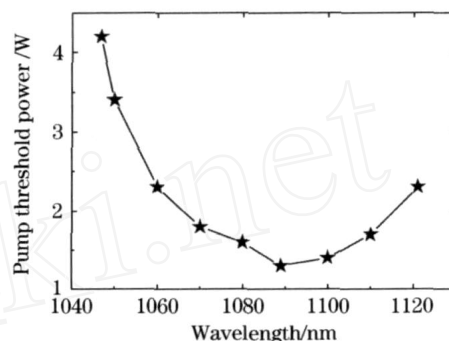
图 4 不同调谐波长处的入纤抽运阈值功率
