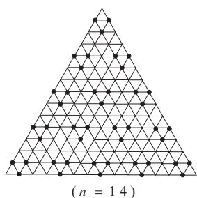
图 4 T(n = 4k + 2)(k = 6m + 3) 的奇数势偶等价覆盖
