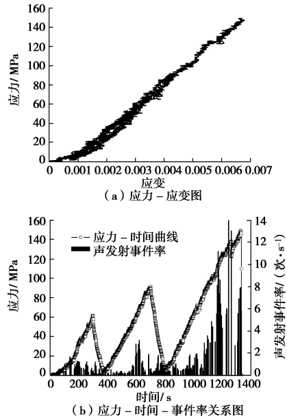
图6 灰岩加卸载试验结果图
