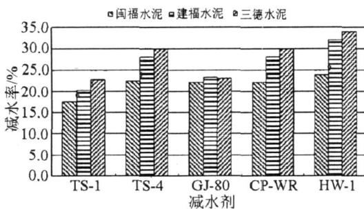
图 2 减水剂在 3 种水泥中的减水率
