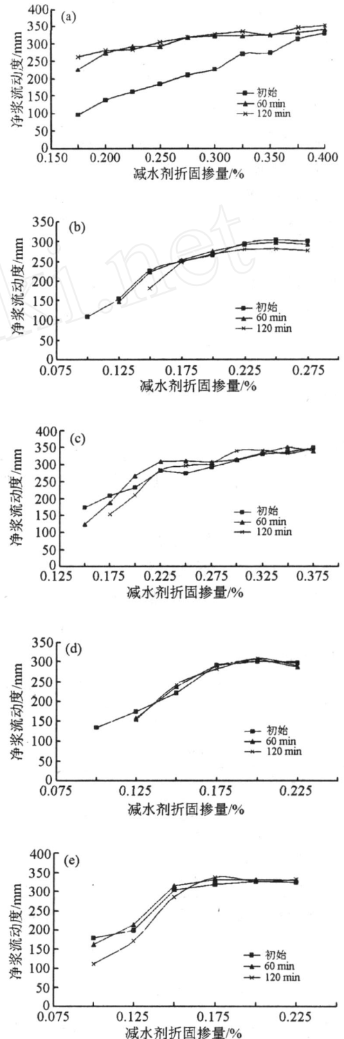
图 1 水泥净浆流动度试验结果
