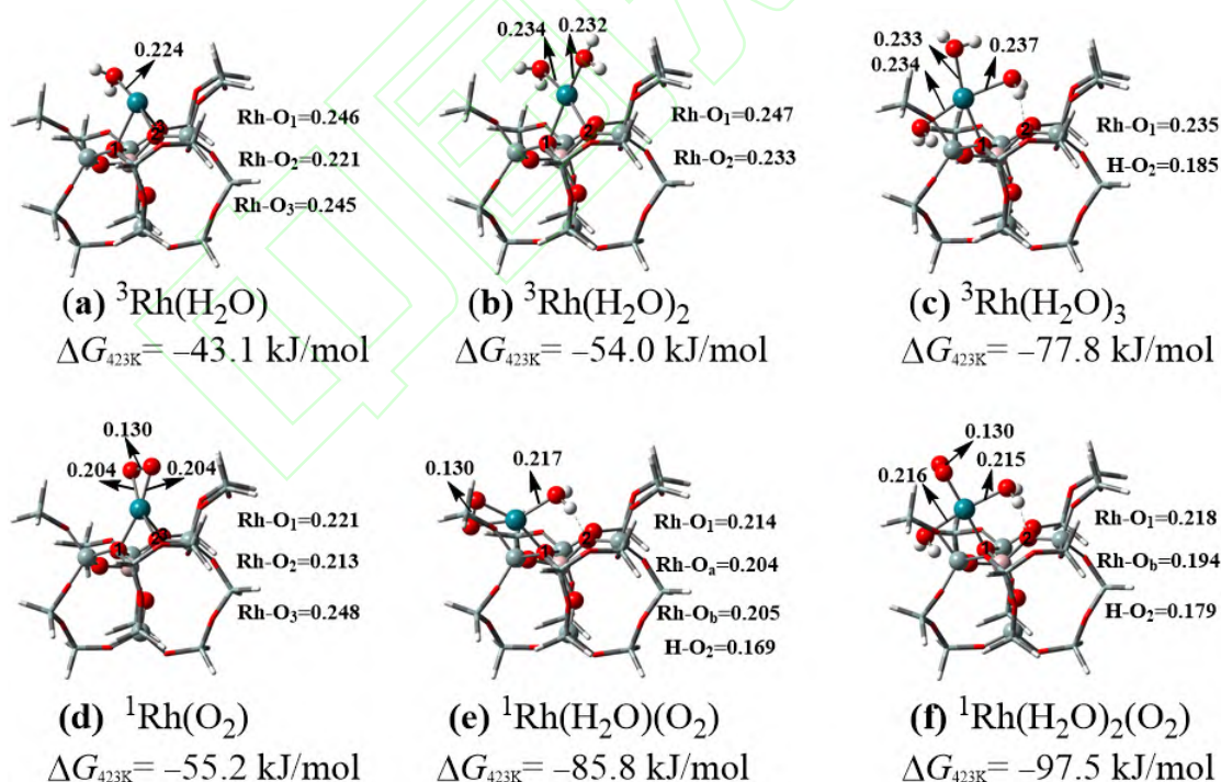
图 2 H 2 O 与 O 2 在 Rh-ZSM-5 上的吸附构型和吸附自由能 (键长单位 nm)
