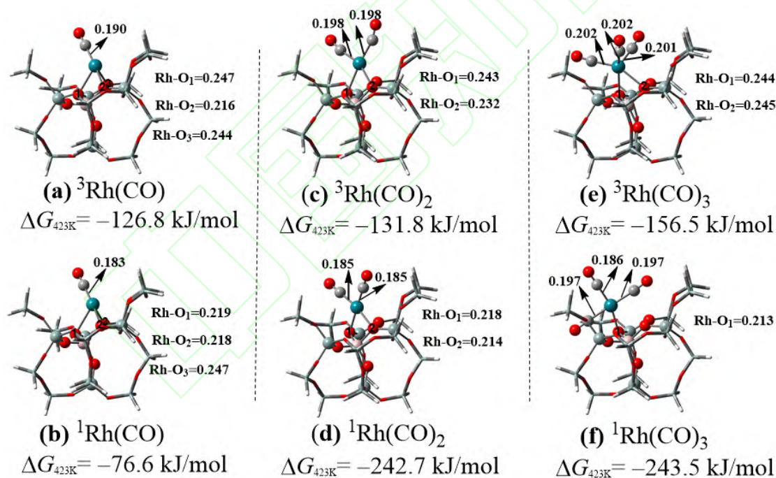
图 3 CO 在 Rh-ZSM-5 上的吸附构型和吸附自由能(键长单位 nm)
