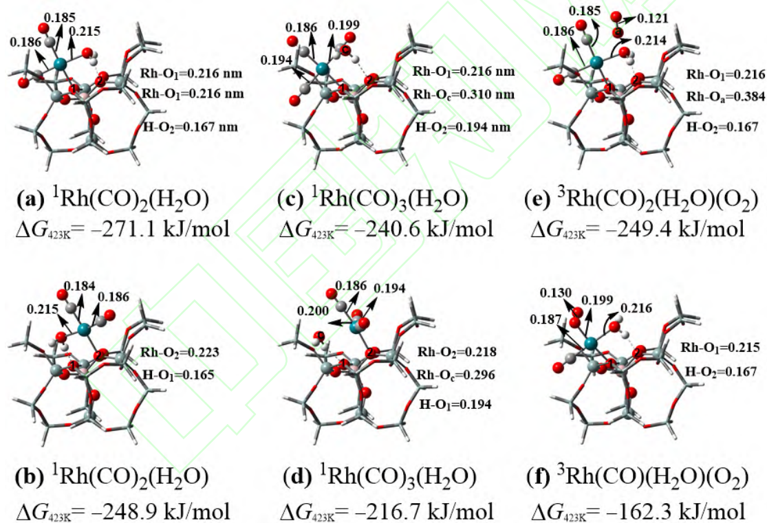
图 4 CO、H 2 O 和 O 2 在 Rh-ZSM-5 上的共吸附构型和吸附自由能(键长单位 nm)
