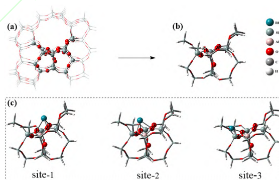
图 1 ZSM-5 簇模型(a) ZSM-5; (b) ZSM-5 的 18T 簇模型; (c) \text{Rh}^+ 在 ZSM-5 内可能吸附位点的构型
