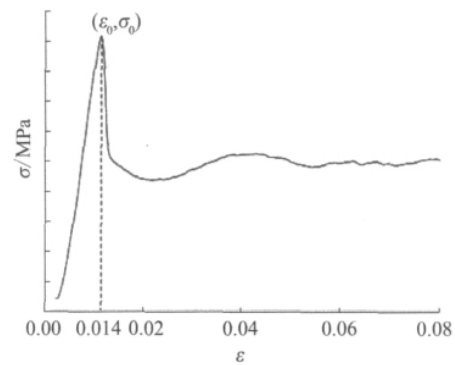
图 5 芯材抗压应力-应变图 Fig. 5 Concrete stress-strain diagram
