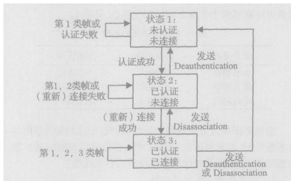
图 1 IEEE 802.11 状态图
