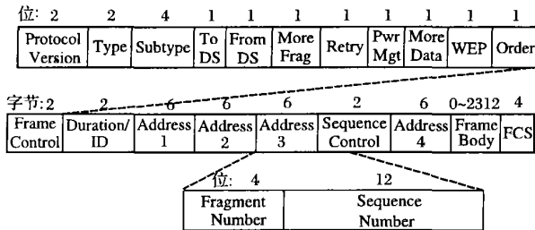
图 3 IEEE 802 11 的 MAC 帧结构
