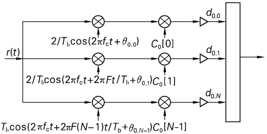
图 2 MG-CDMA 的接收机框图
