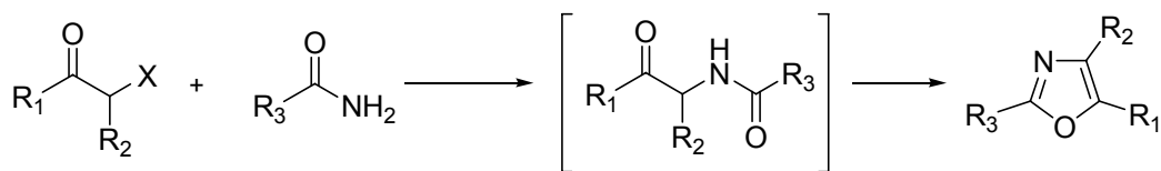
图 1-7 利用 Hantzsch 条件用 \alpha -卤代酮与酰胺合成多取代噁唑
