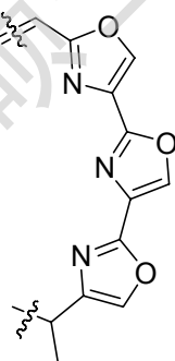
图 1-9 Ulapualide A 片段
