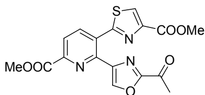
图 1-8 dimethyl sulfomycinamate
