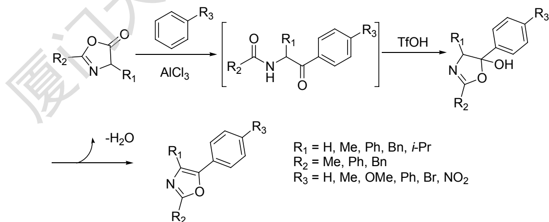
图 1-6 由噁唑酮经过 Friedel-Crafts/Robison-Gabriel 反应合成 2,4,5-三取代噁唑
