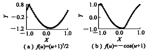
图 2 计算结果 ( \Delta x = 0.05, t = 1.5/\pi^2 )
