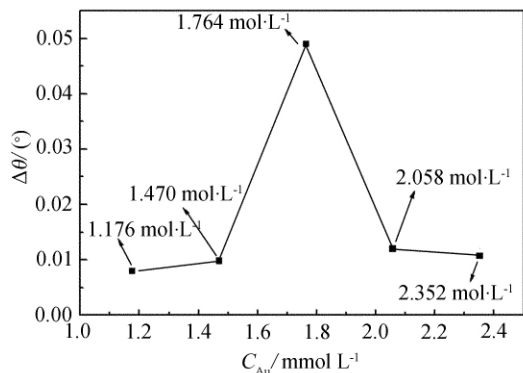
图 4 不同浓度金液湿化学镀金基底在 2% (by volume) 酒精中的 SPR 响应
