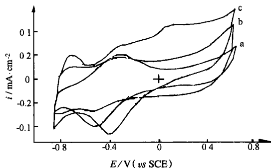
图 1 PPDMAE 在不同 pH 值的 \text{NaNO}_3 溶液中的循环伏安图
