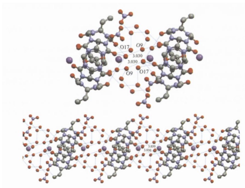
图 3 (\text{CyH})_2\text{Q}[6]-\text{Na}(\text{I}) “分子胶囊”构成的一维超分子链
