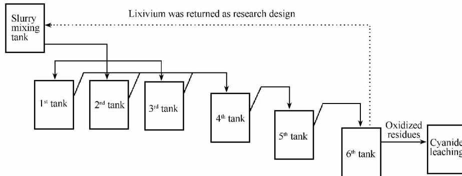
图 1. 连续生物预氧化基本流程
