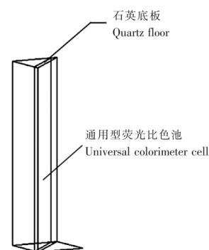
图1 多用途荧光比色皿的示意图
