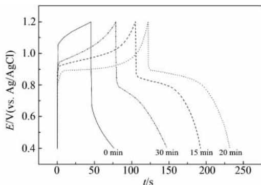
图 7 8 mA·cm 2 电流密度下不同氧气等离子体处理时间石墨电极 VO 2+ /VO 2 + 电对第 10 周的充放电曲线
