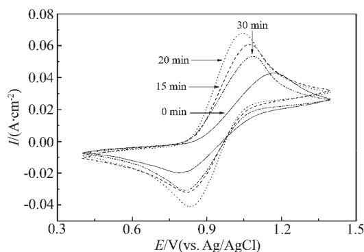
图 5 不同氧气等离子体处理时间的石墨电极在 2 mol·L -1 VOSO 4 + 2 mol·L -1 H 2 SO 4 溶液中的循环伏安曲线(扫速 10 mV·s -1 ) Fig. 5 CV curves of untreated and oxygen plasma treated graphite plate electrodes for different time, recorded at 10 mV·s -1 in 2 mol·L -1 VOSO 4 + 2 mol·L -1 H 2 SO 4 solution
