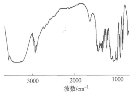
图 1 苦楝素的红外光谱图
