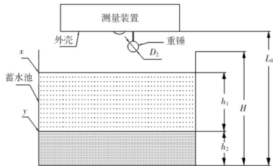
图 3 水深水位测量装置的测量原理图
