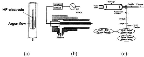
图 10 各种单针电极式等离子体射流发生器
