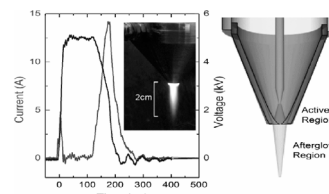
图 5 便携的纳秒脉冲等离子体射流发生器
