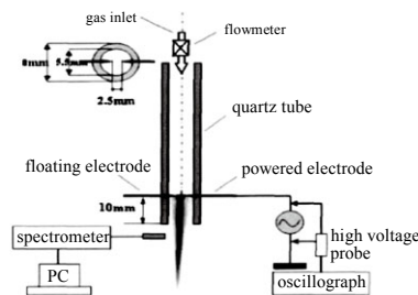
图 9 悬浮电极式大气压等离子体射流发生器
