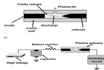
图 4 腔体放电产生等离子体射流发生装置
