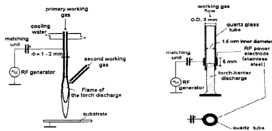
(a) 大气压炬放电 (b) 大气压阻挡炬放电
