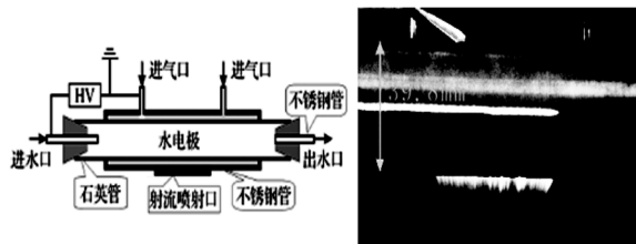
图 11 同轴电极等离子体射流发生器
