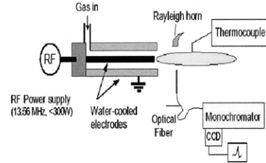
图 12 射频等离子体射流装置
