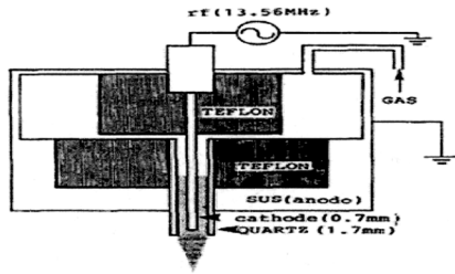
图 1 日本东京工业学院发明的等离子体发生器
