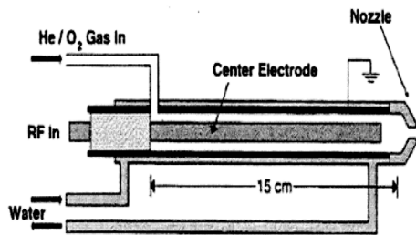
图 2 Los Alamos 研制的 APPJ 发生器
