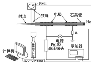
图 8 环-环式电极等离子体射流发生器
