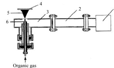
图 13 微波源激励产生等离子体射流的装置
