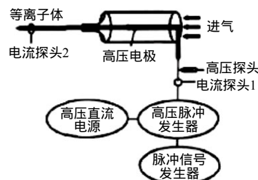
图 15 单电极大气压低温等离子体射流装置
