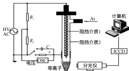
图 7 双层介质阻挡等离子体射流发生装置
