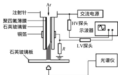
图 6 中空针状电极的等离子体射流发生器
