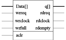
图2 LPM-FIFO-DC 元件符号图
