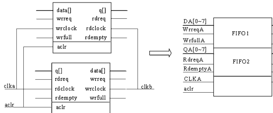
图3 双通道FIFO 存储器模块原理图
