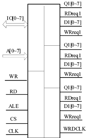
图 5 多路逻辑端口图形符号
