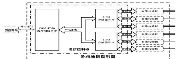
图1 测控系统框图
