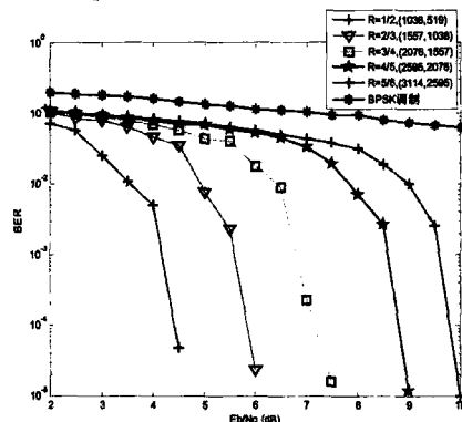
图 4 RC QC-LDPC 编码在 NSVG 水声信道中的 BER 曲线
