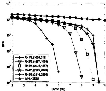
图 3 RC QC-LDPC 编码在 ISVG 水声信道中的 BER 曲线
