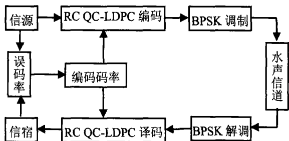
图 1 水声自适应信道编码通信原理图
