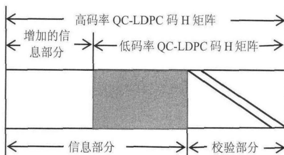
图 2 扩展信息位方法示意图
